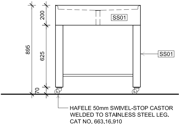
03 ELEVATION 1:20
