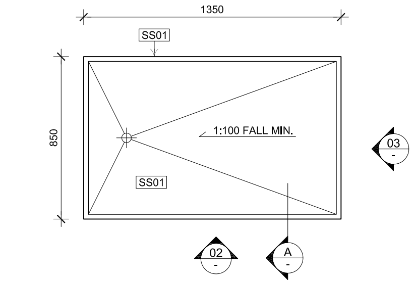
01 TOUCH TABLE PLAN 1:20
