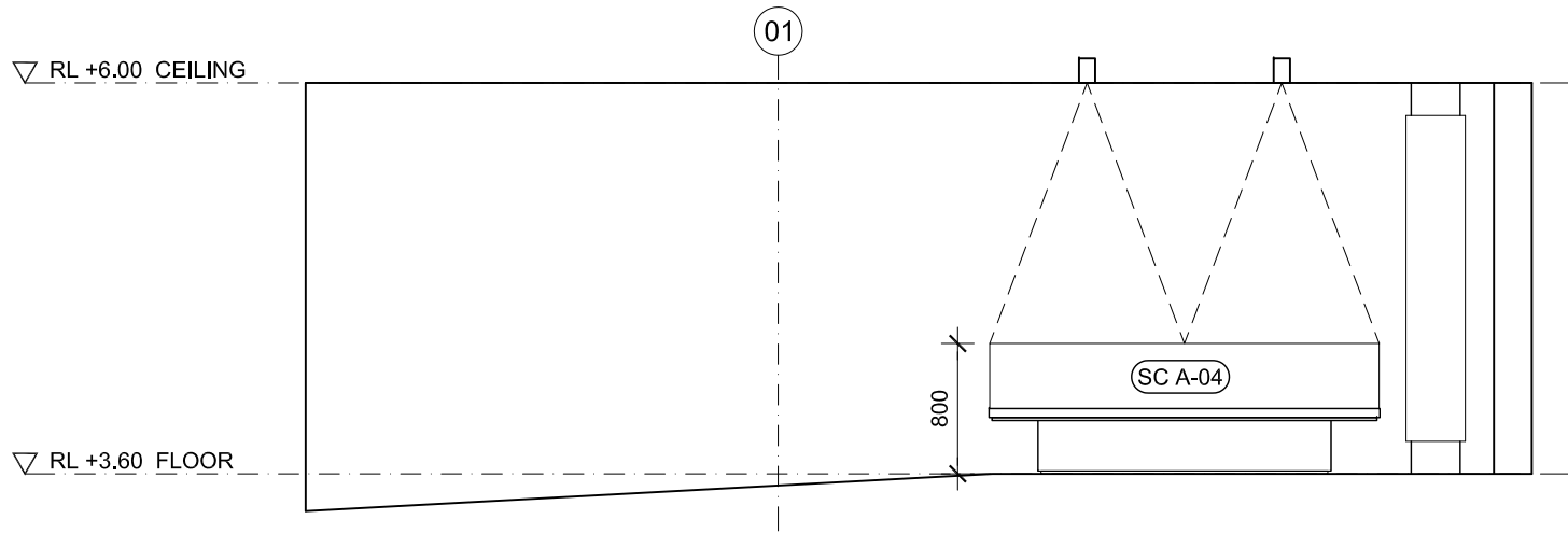
01 ELEVATION A1.02 1:100
