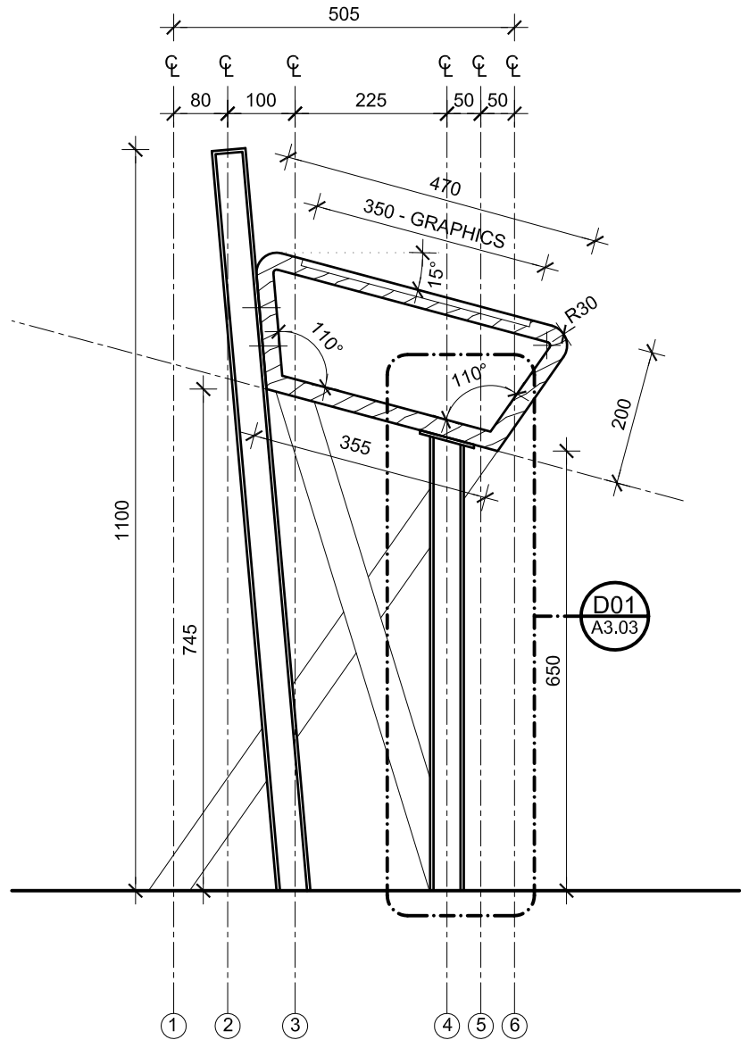
DD SECTION A3.10 1:10
