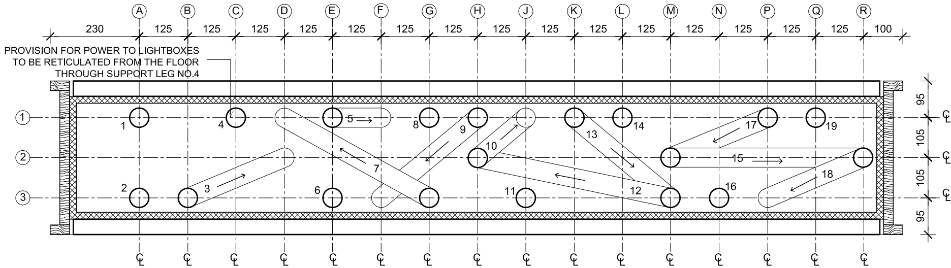
01 ANGLED LEG SETOUT PLAN - 1:10
