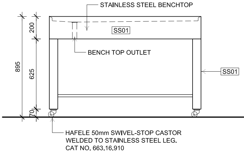
02 ELEVATION 1:20
