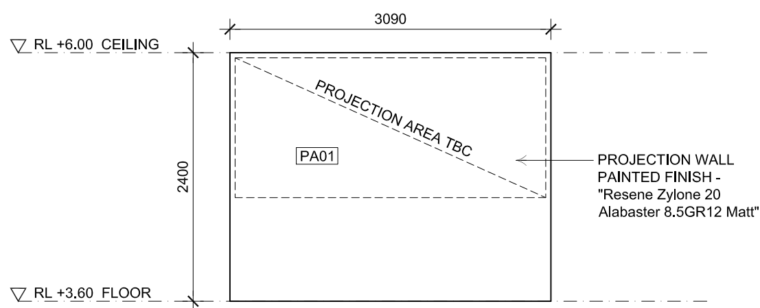
02 ELEVATION A1.02 1:100
