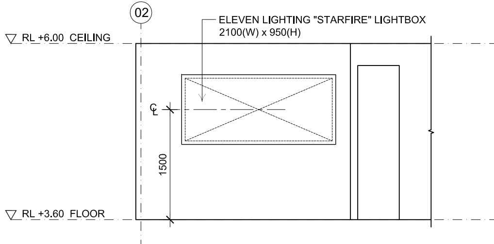
04 ELEVATION A1.02 1:100
