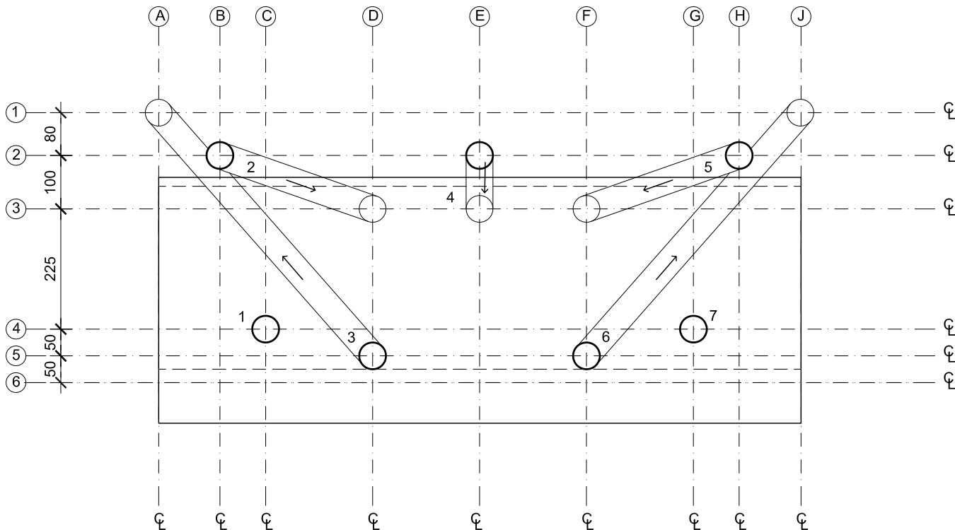
05 ANGLED LEG SETOUT PLAN - 1:10
