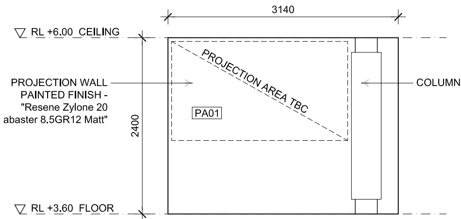
03 ELEVATION A1.02 1:100
