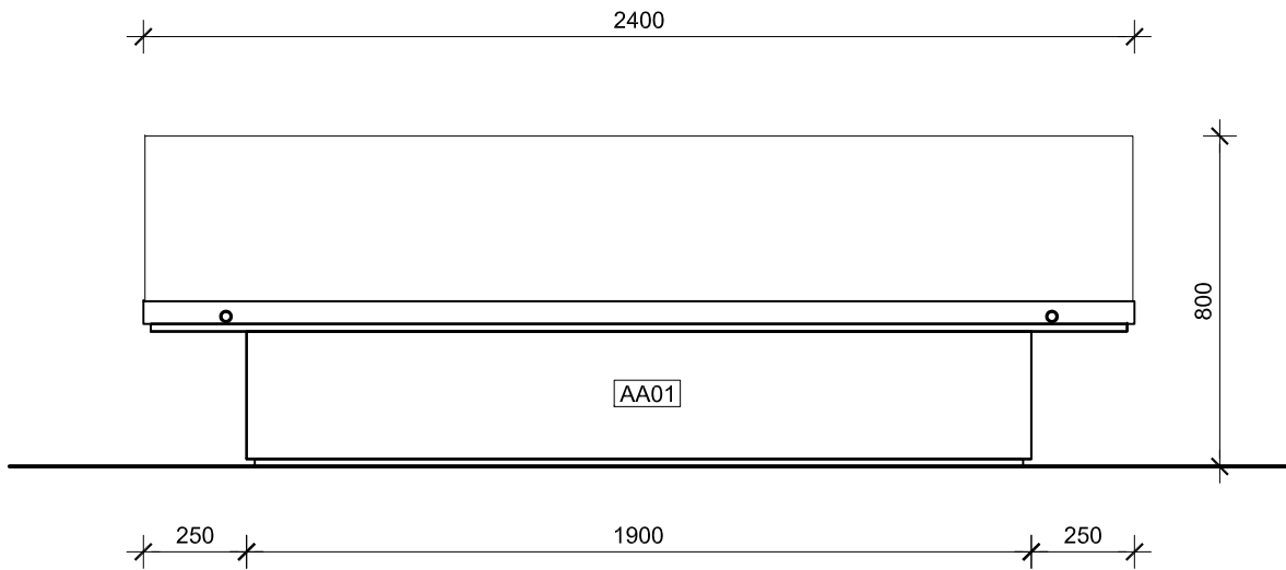
02 ELEVATION 1:20
