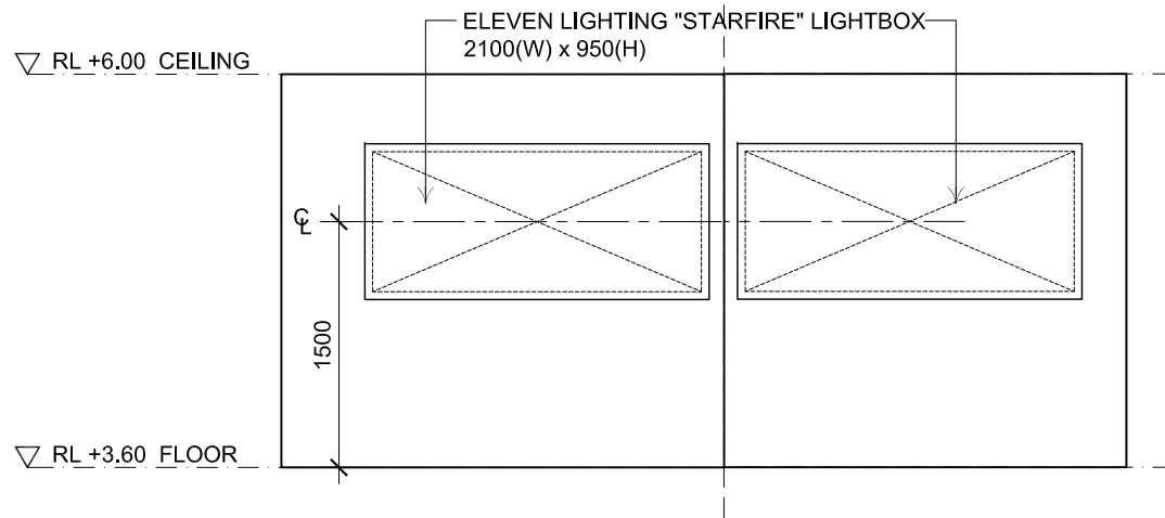
06 ELEVATION A1.02 1:100
