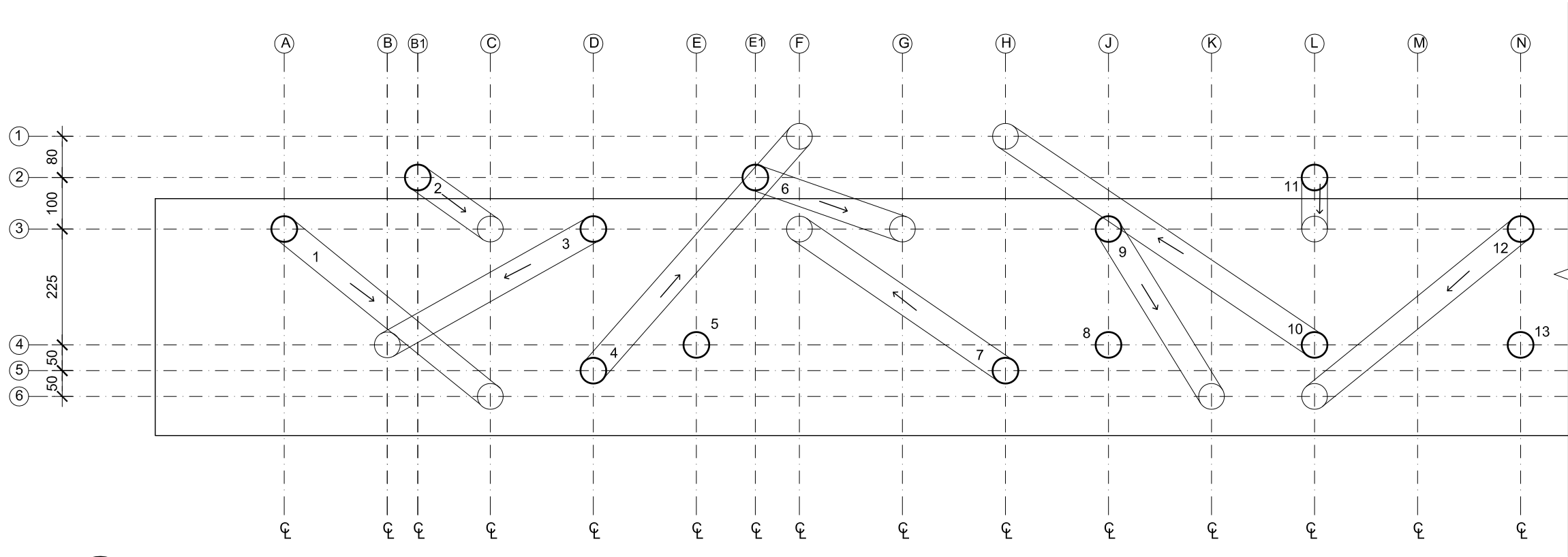
01 ANGLED LEG SETOUT PLAN - PART 1 - 1:10
