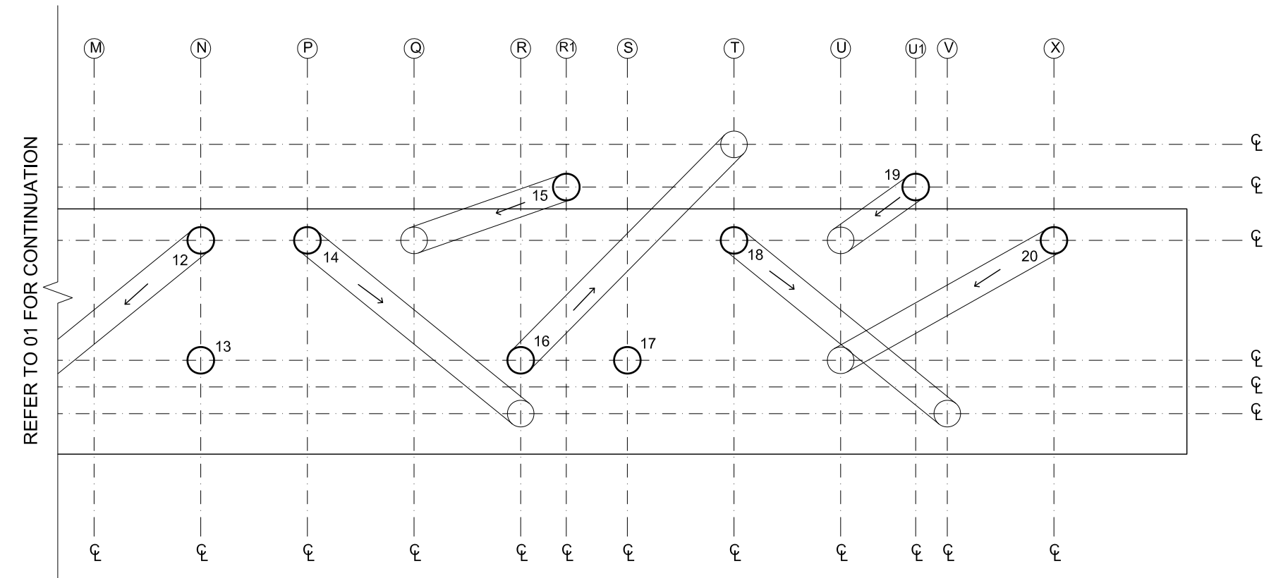
02 ANGLED LEG SETOUT PLAN - PART 2 - 1:10
